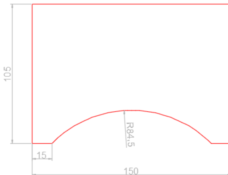
Rysunek 1 Rzut z góry elementu. Uwaga! Wymiary podano w cm.
